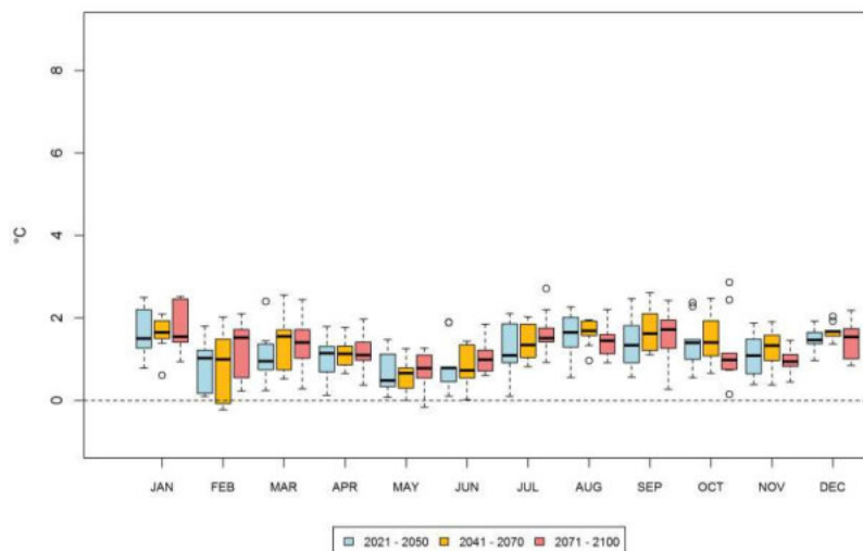
Abb. A 5: Änderung der langjährigen monatlichen Mitteltemperaturen in Kaiserslautern (RCP 2.6)
