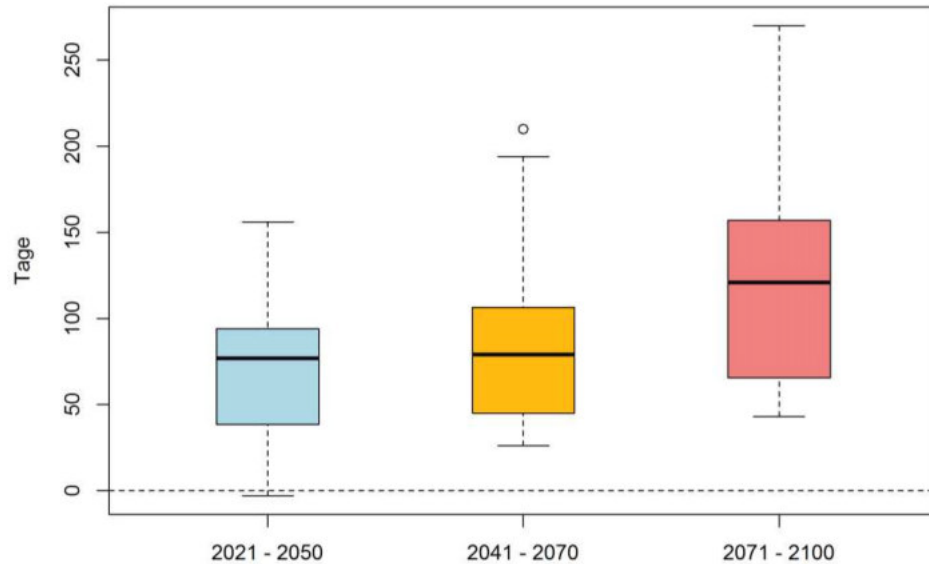
Abb. A 21: Änderung der Auftrittshäufigkeit von Niederschlagsereignissen mit N \geq 20 mm/d innerhalb des jeweiligen 30-jährigen Zeitraumes in Kaiserlautern, Szenario RCP 8.5
