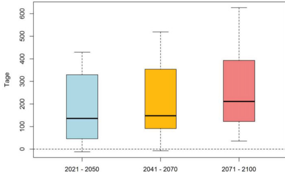
Abb. A 18: Änderung der Auftrittshäufigkeit von Niederschlagsereignissen mit N \geq 10 mm/d innerhalb des jeweiligen 30-jährigen Zeitraumes in Kaiserslautern, Szenario RCP 8.5
