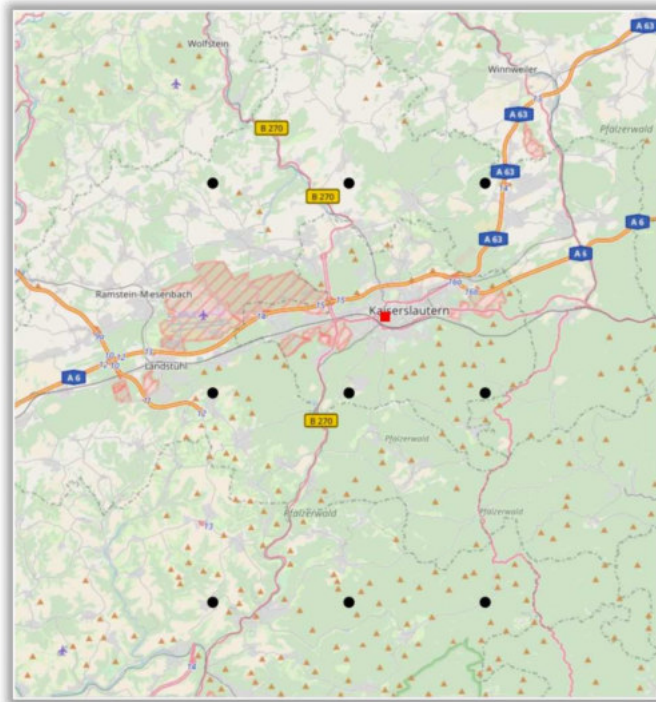
Abb. A 1: Für die Analyse des Klimawandels in Kaiserslautern ausgewählte Gitterpunkte aus dem EURO-CORDEX-Modellgitter ( Hintergrund: © OpenStreetMap contributors, Open Database www.opendatacommons.org/licenses/odbl )
