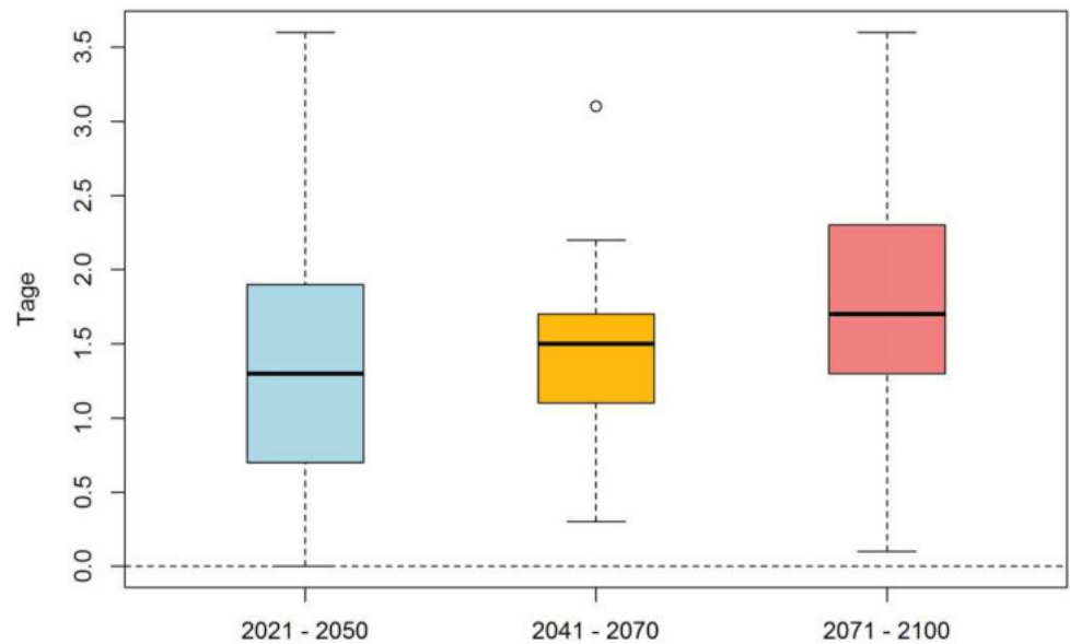
Abb. A 7: Änderung der Länge von Hitzeperioden (aufeinanderfolgende Tage mit T_{max} \geq 30 \text{ °C} ) in Kaiserslautern. Szenario RCP 2.6
