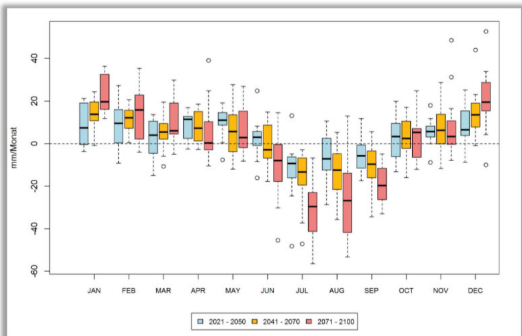
Abb. 21: Änderung der langjährigen mittleren monatlichen klimatischen Wasserbilanz in Kaiserslautern, Szenario RCP 8.5
